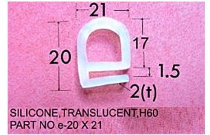
YES346 e 20x21
