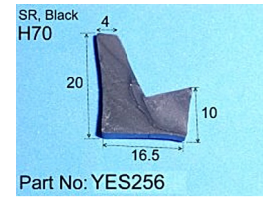
YES256 (if EPDM YEC172)
